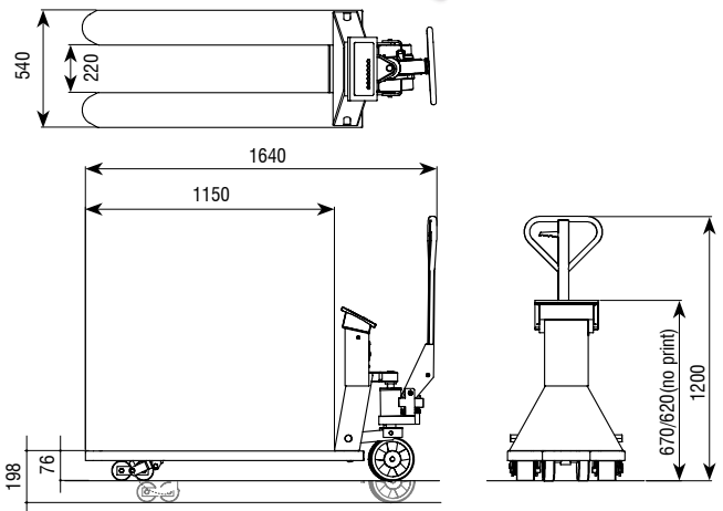
Transpaleta ARXLED Wide (para palés americanos)
